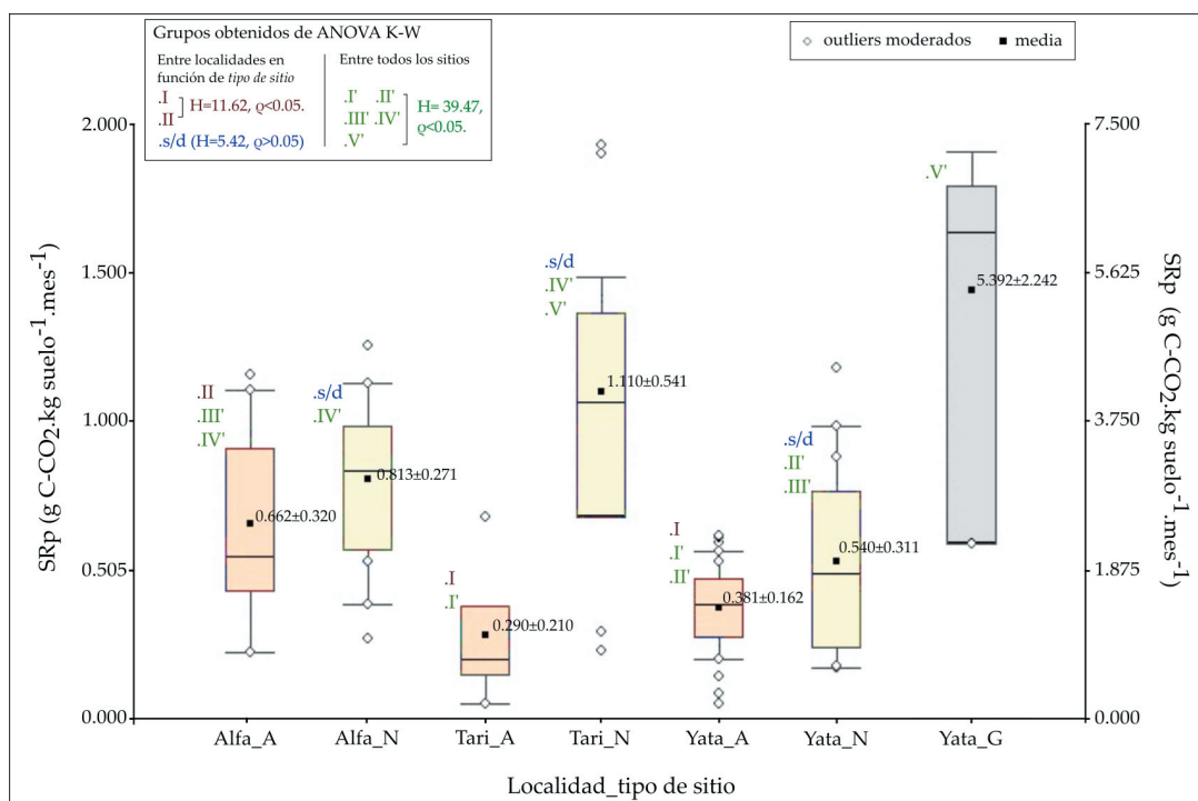
Figura 3. Gráficos de cajas de las SRp medidos por localidad y tipo de sitio, con información de los grupos resultantes de las pruebas post-hoc ANOVA (Kruskal-Wallis), que comparan localidades por tipo de sitio y en todos los sitios analizados (los sitios híbridos, de dunas naturales y naturales degradados se categorizaron como 'naturales' para estos análisis). Las cajas representan el 68% de los datos (1 DE), y la línea central indica la mediana. El eje vertical de la derecha corresponde al sitio ganadero Yatagán. Se reportan los valores de media y desviación estándar para cada caso, excluyendo valores outliers. Tari_A=sitios agrícolas de Tari; Tari_N=sitios naturales de Tari; Yata_A=sitios agrícolas de Yatagán; Yata_N=sitios naturales de Yatagán; Yata_G=sitio ganadero de Yatagán; Alfa_A=sitios agrícolas de Alfalfares; Alfa_N=sitios naturales de Alfalfares. Las clases asignadas a más de un grupo dentro del mismo análisis indican limitaciones de la prueba estadística.
