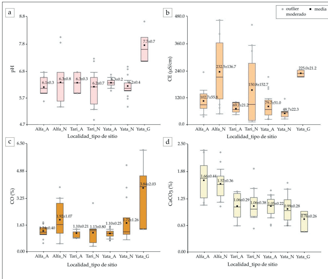
Figura 4. Gráfico de cajas de las propiedades fisicoquímicas del suelo por localidad y tipo de sitio. a) pH. b) CE (conductividad eléctrica, \mu\text{S}/\text{cm} ). c) CO (carbono orgánico, %). d) CaCO 3 (%). Las cajas representan el 68% de los datos (1 DE) y la línea horizontal central de la caja representa la mediana. Se excluyen los valores extremos de cada propiedad y en cada caso se informa el valor de la media y la desviación estándar.
