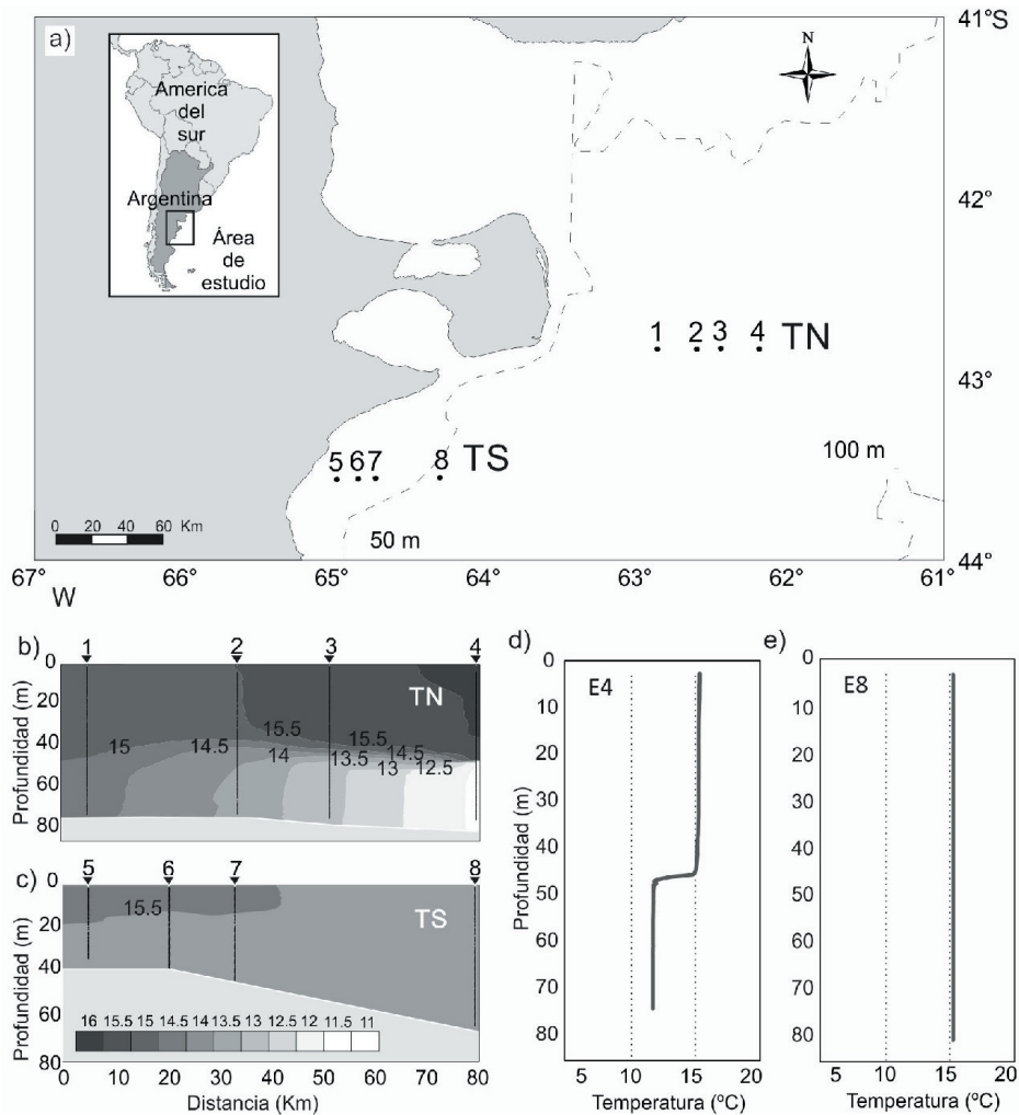
Figura 1 a) Distribución espacial de las estaciones estudiadas, transecta norte (TN), transecta sur (TS). b) Perfil vertical de temperatura (°C) en la TN. c) Perfil vertical de temperatura en la TS. d) Perfil vertical de temperatura en la estación 4 (E4) de la TN. e) Perfil vertical de temperatura en la estación 8 (E8) de la TS.
