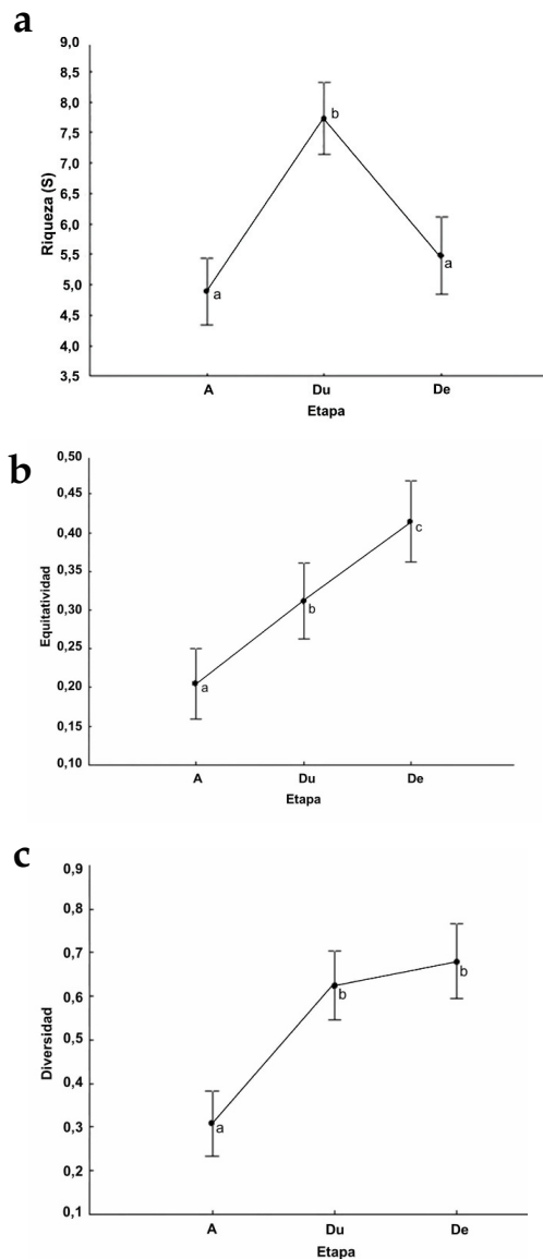
Figura 3. Variación temporal de la a) riqueza, b) equitatividad y c) diversidad en los sitios de estudio [sitio 1 (1200 m al sur de efluente), sitio 2 (8000 m al norte) y sitio 3 (9000 m al norte del efluente)], en las distintas etapas [antes de la construcción del emisario (A), durante la construcción (Du) y posterior a la construcción (De)]. El punto medio indica la media y el largo de las barras el 0.95 de los intervalos de confianza. Las letras indican diferencias significativas ( P < 0.01 ). Cuando la interacción S*E no resultó significativa, los datos correspondientes a los sitios fueron agrupados.
