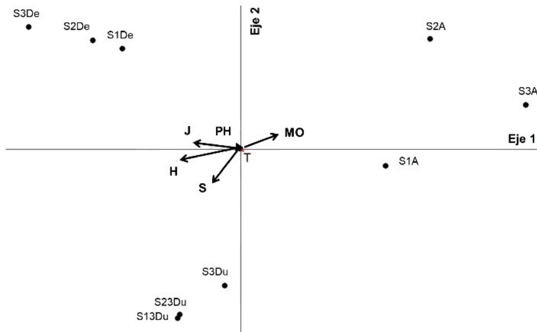
Figura 4. Análisis de componentes principales (ACP) integrando las variables biológicas (S: riqueza, J: equitatividad y H: diversidad) y las variables ambientales (T: temperatura, MOT: materia orgánica total y pH) en los tres sitios de muestreo durante las diferentes etapas [antes de la construcción del emisario (A), durante la construcción (Du) y posterior a la construcción (De)].
